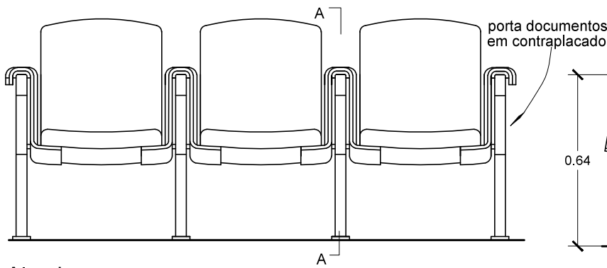
Alçado Escala 1/20
