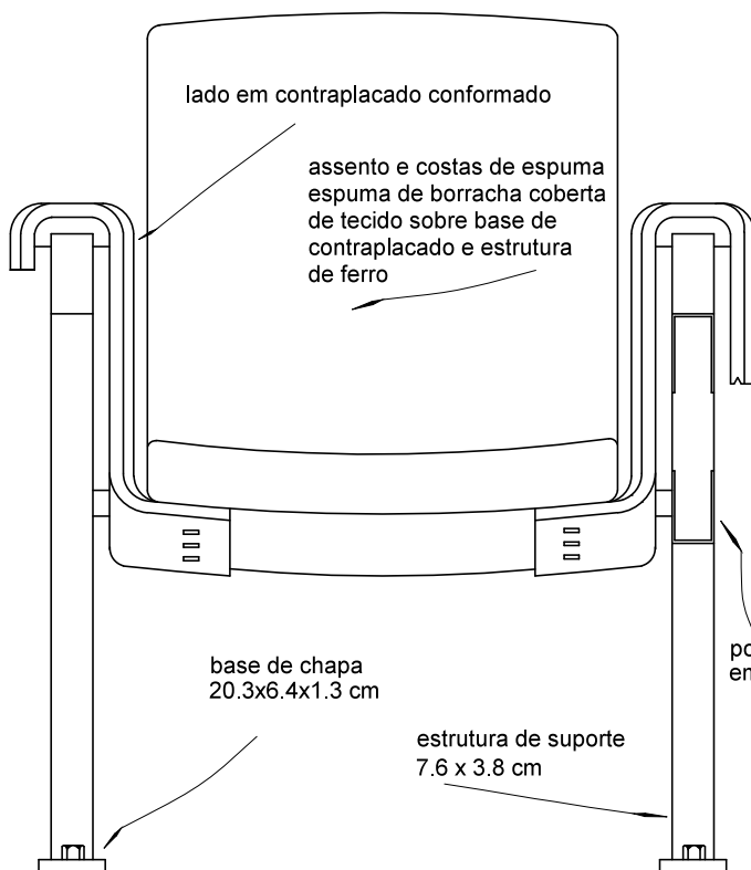
Alçado Escala 1/8
