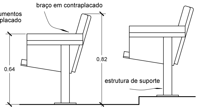
Alçado Escala 1/20
