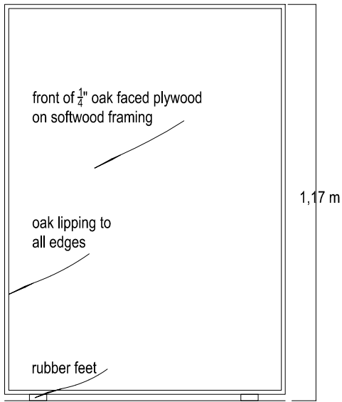
ELEVAÇÃO FRONTAL escala 1/15
