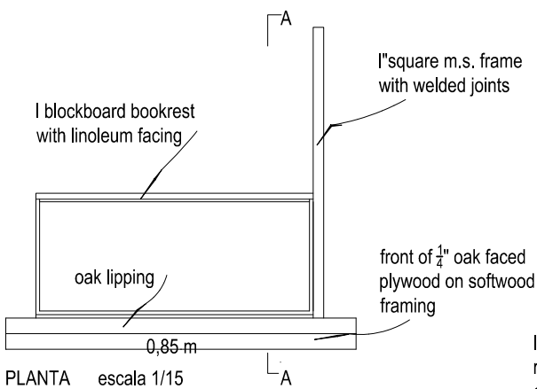
PLANTA escala 1/15
