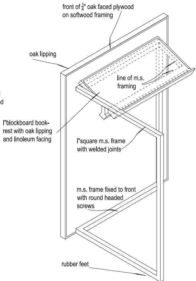
VISTA ISOMÉTRICA
