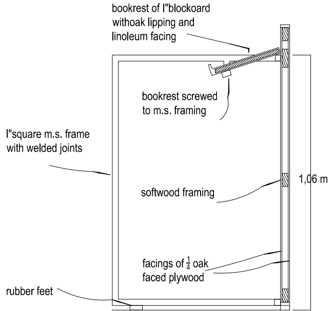
SECÇÃO A - A escala 1/15
