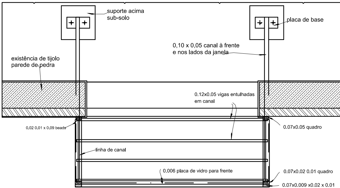
PLANO DA JANELA EM BALANÇO escala 0.01=0.30
