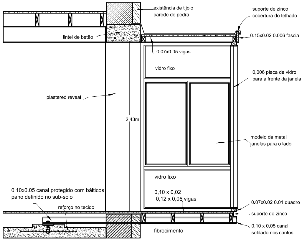
SECÇÃO ATRAVÉS DA JANELA EM BALANÇO - ESCALA 0,01=0,30
