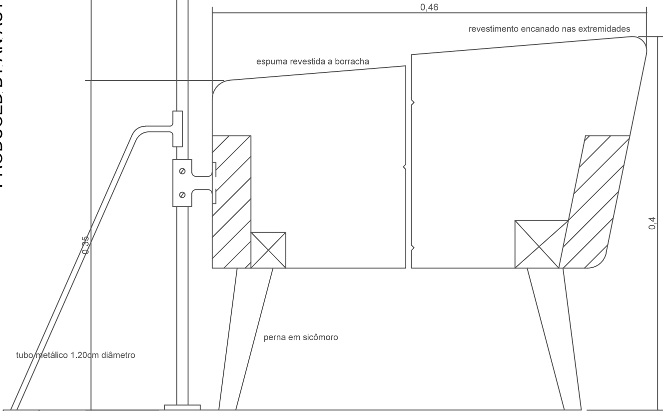
secção pela prateleira escala. 1/2
