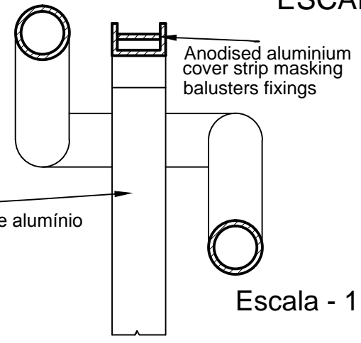
Corte B
